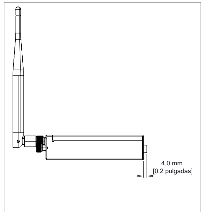
Vista lateral
